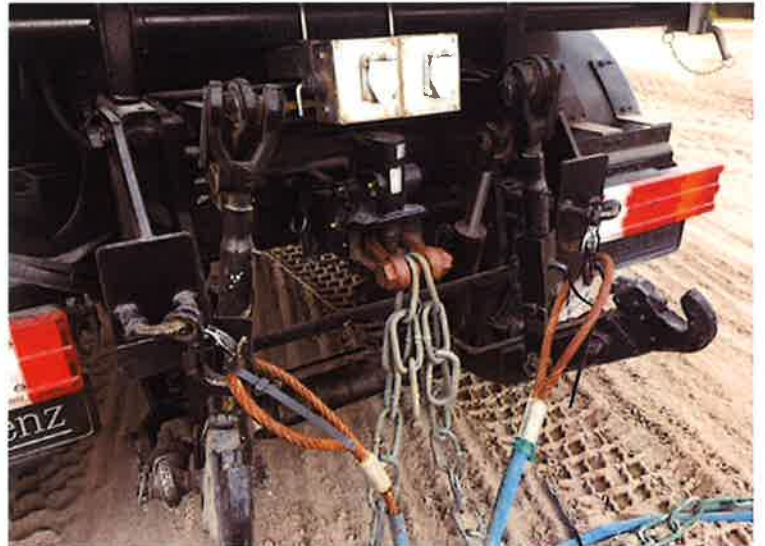
3箇所牽引しているが、真ん中のチェーンのみでも牽引可能
