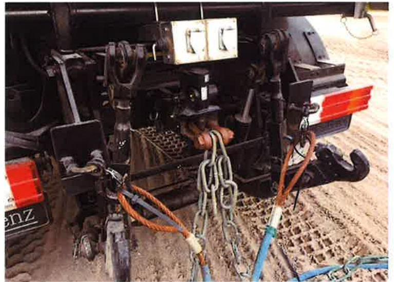
3箇所で牽引しているが、真ん中のチェーンのみでも牽引可能
