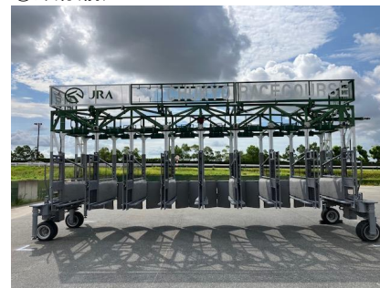
①外観(前)
